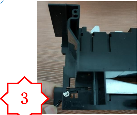
③ 装入 MC2447 组件
