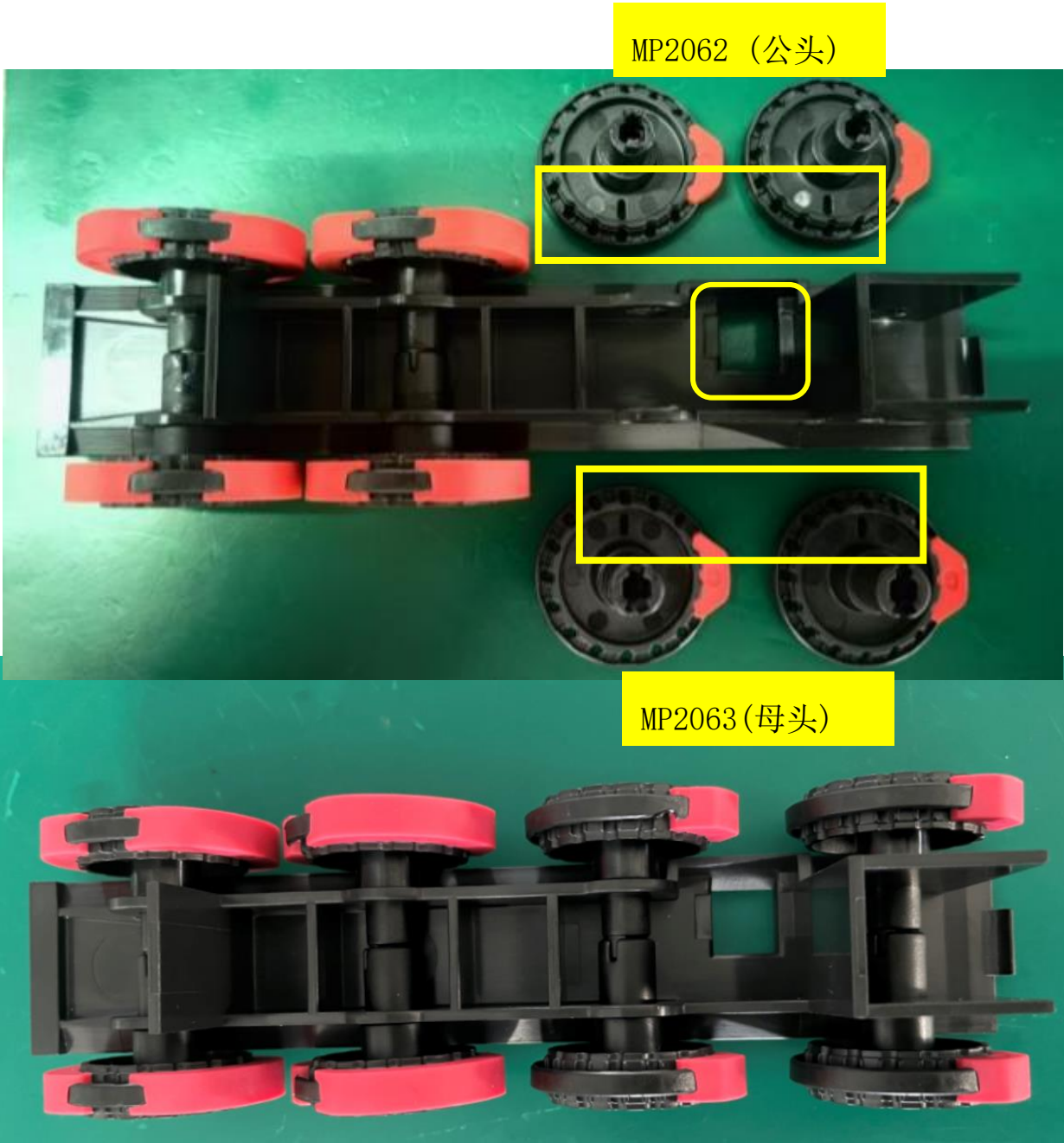
图 1，将两个 MP02062 和 MP2063 分别装配在导光柱方孔方向，按照图示方向正确装配，黄色方框内条形方形小槽方向相对！
