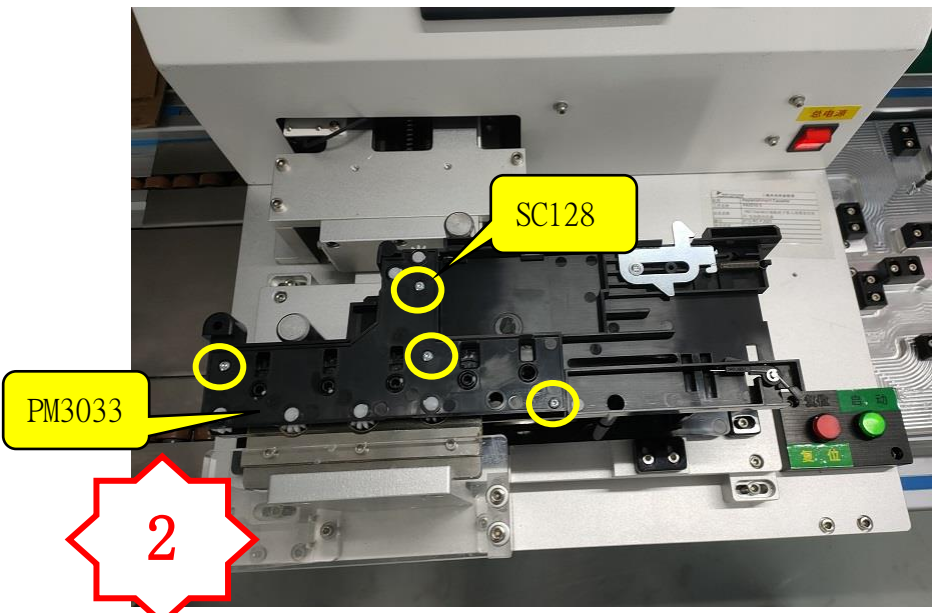
2. 装入已经刷了油的 PM3033，和打 4 颗 SC128
