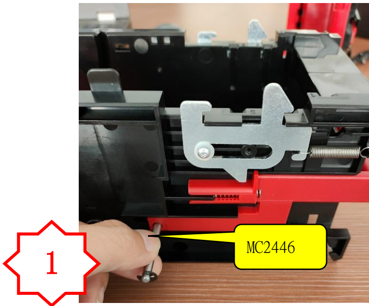
1. 将 MC2446 组件穿过红色组件的孔 到另一侧 PM3034 的孔
