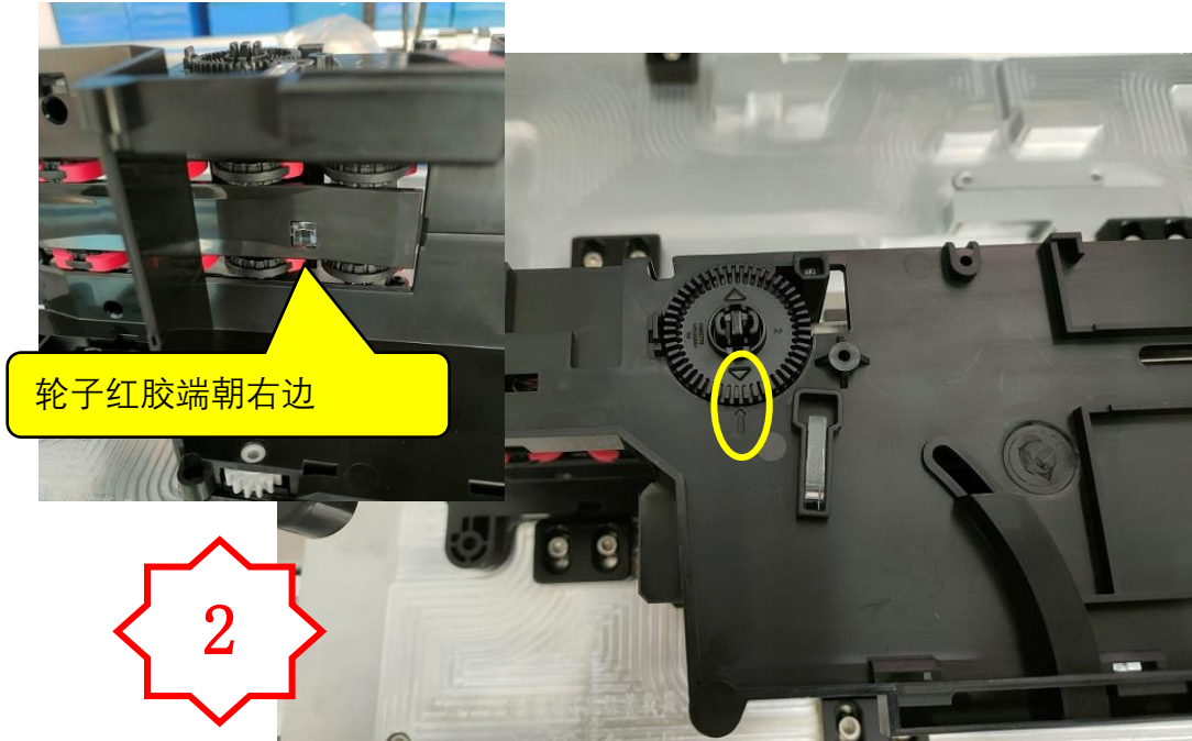
2. 检查轮子红胶朝右，两箭头对准后将齿轮压到位！
