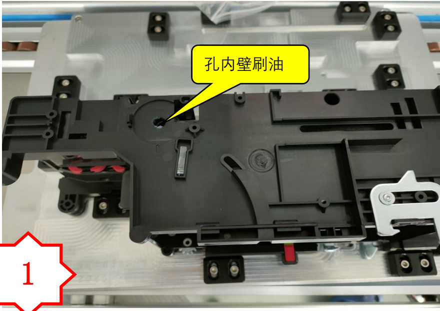
1. 在组件的孔内刷少量 NYE368F 润滑油脂，油脂可见不堆积。
