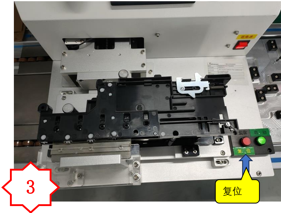
3. 按复位按钮，取出半成品进行翻转放到倍速链固定治具上
