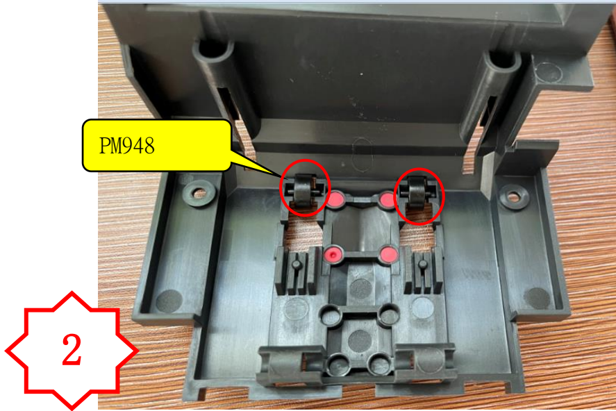
2. 如上图装入两个 PM948
