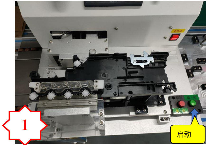
1. 将半成品放到设备上，按下绿色启动按钮
