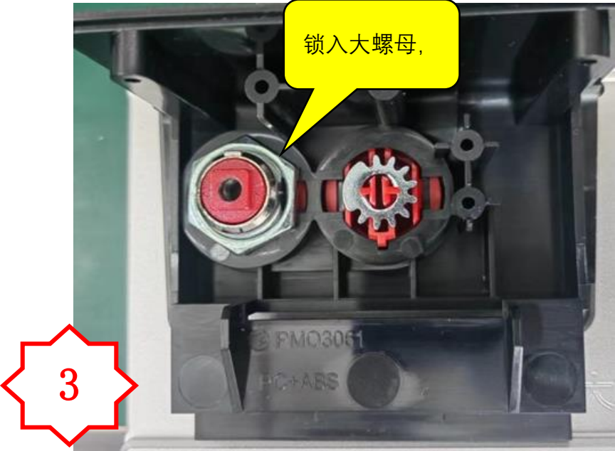
3. 螺母②锯齿面朝下装入, 然后锁紧。
