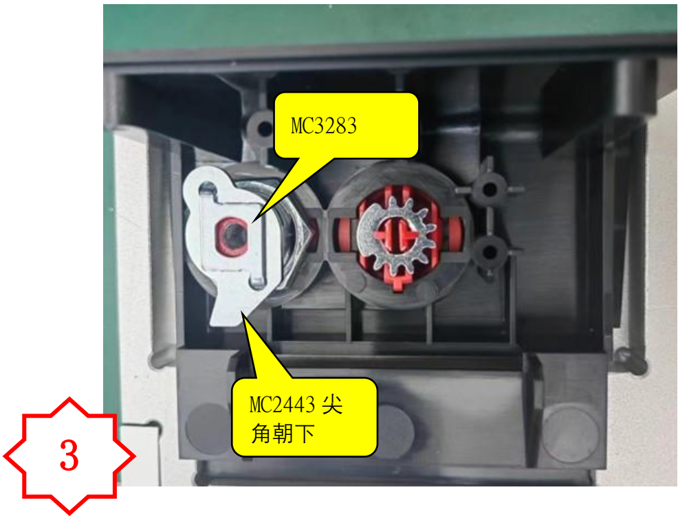
3. 按图示方向装入 MC2443+MC3283.
