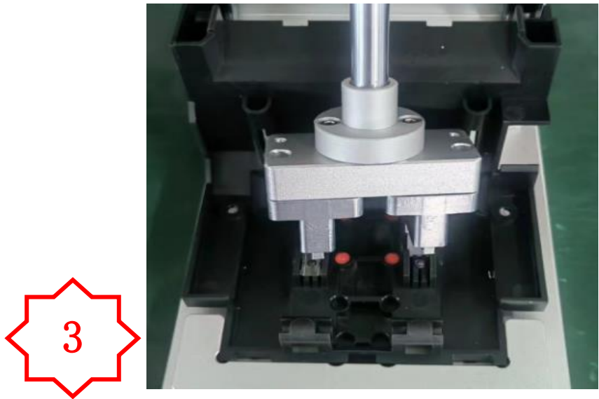
3. 将 PM3038+SP172 放入治具，确认装配到位后再进行压合。
