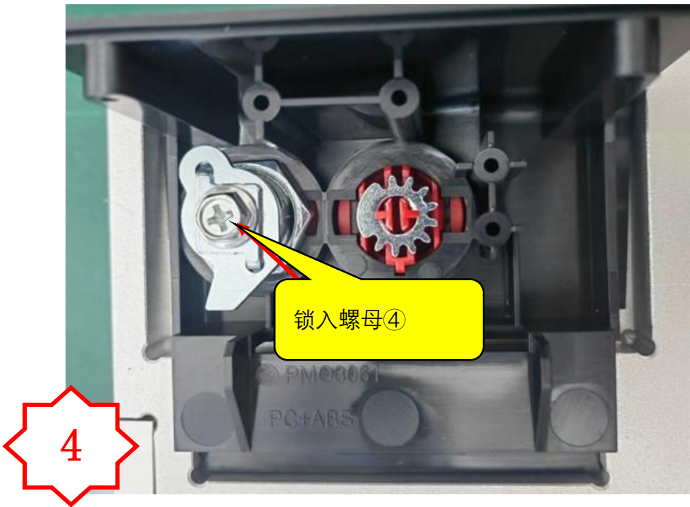
4. 检查 MC2443+MC3283 装配到位后锁入螺母④
