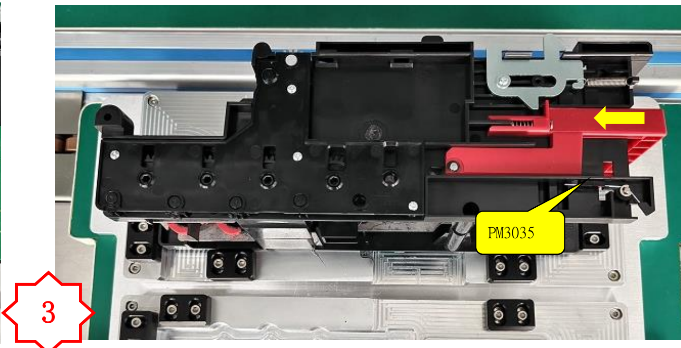
3. 将 PM3034 推到底后复位，PM3035 可弹起卡住 PM3034
