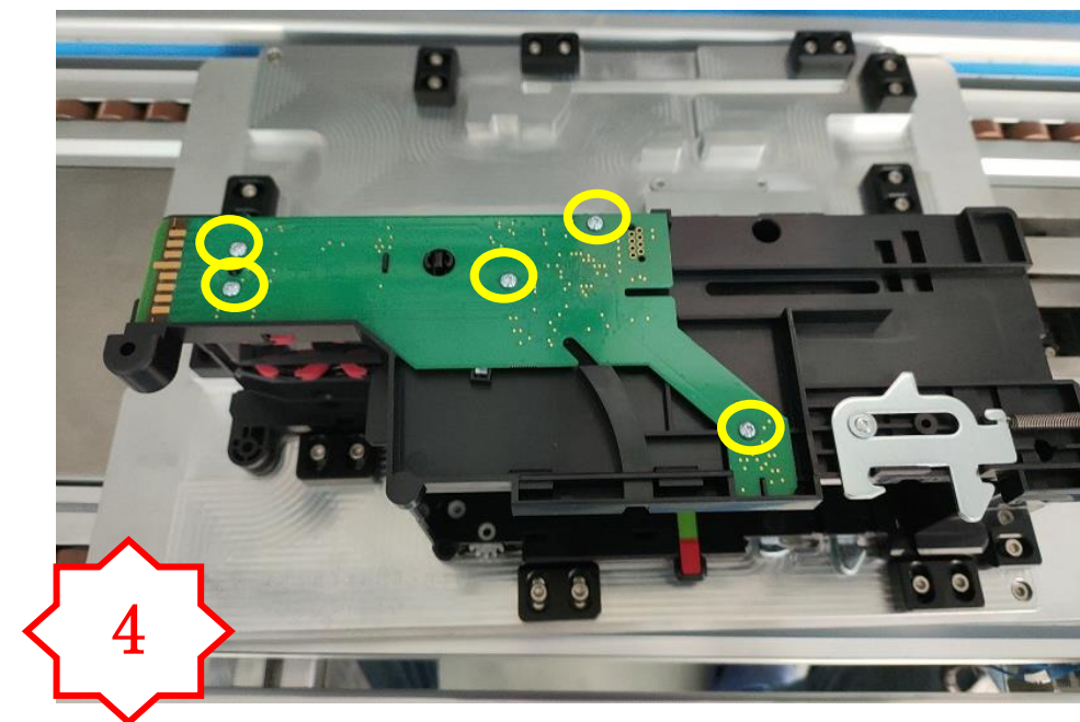
4. 打 5 个 SC128 螺丝
