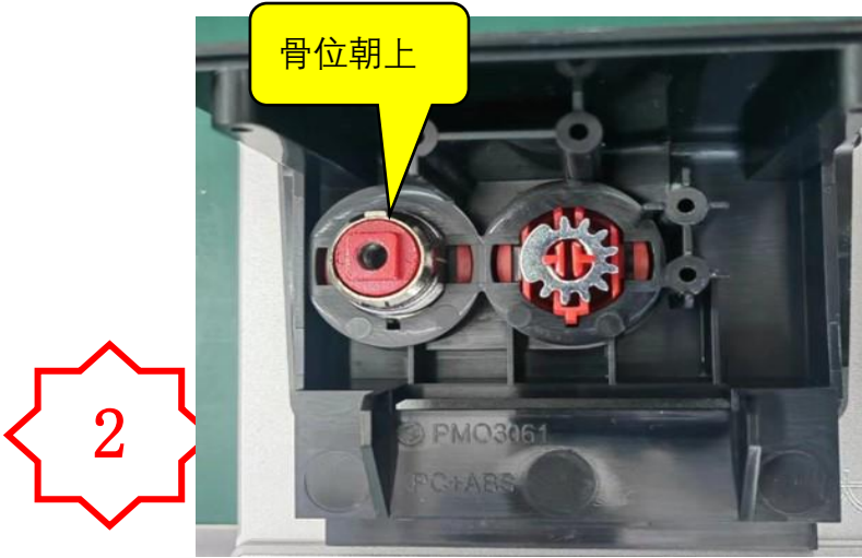
2. 将锁①按图示方向装入, 锁的红色长柄朝箭头头位, 放进治具, 检查骨位在螺丝柱方向。
