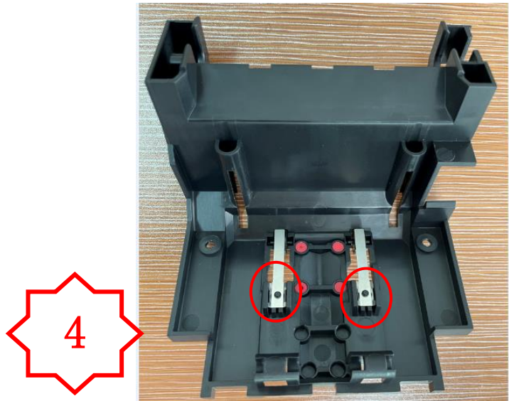
4. 检查 SP172 平的一面朝下，压紧到 PM3038 对应柱上。
