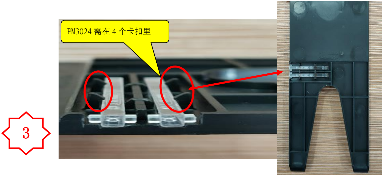
3. 检查装到位后，PM3024 需在 PM2042 的 4 个卡扣里。
