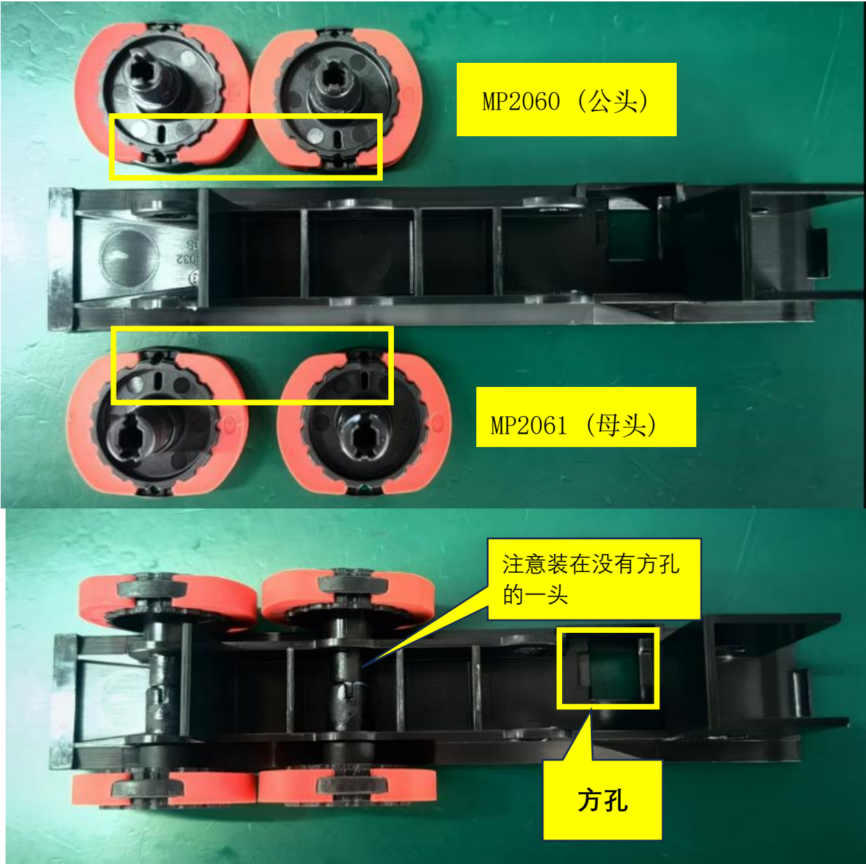
图 1，分别将 2 个 MP2060 和 MP2061 装配在无方孔方向的两个孔，按照图示方向正确装配，黄色方框内条形方形小槽方向相对！
